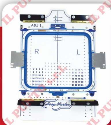
Esempio Attacchi di collegamento Station con telaio 28 x 33 su Station Standard.
